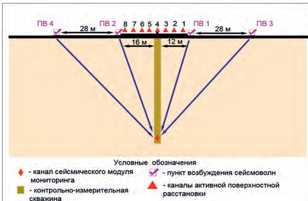
▲ Рис. 2. Система наблюдения при наземно-скважинной съемке.
