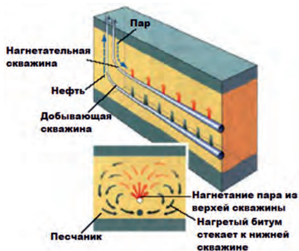
▲ Рис. 1. Схема SAGD (Meyer, R. F., E. Attanasi, 2003).
