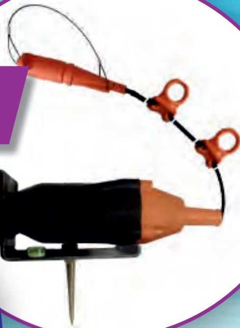
Solo 5-10Hz Горизонтальный геофон, чувствительность 80V / M / S
