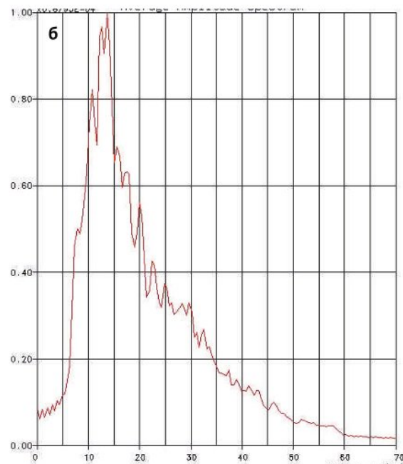
▲ Рис. 5. Сопоставление спектров отражённых волн, зарегистрированных с использованием группы 2-х вибраторов на базе 10 м и 3-х вибраторов на базе 20 м (ПР1, ПВ1051, \Delta F=6-60 Гц, T=24 с, \text{пнак}=6 , начальный скос 200 мс., конечный скос 500 мс., окно анализа 1,5-2,5 с, вне конуса доминирующих поверхностных помех); а – два вибратора на базе 10 м; б – три вибратора на базе 20 м
