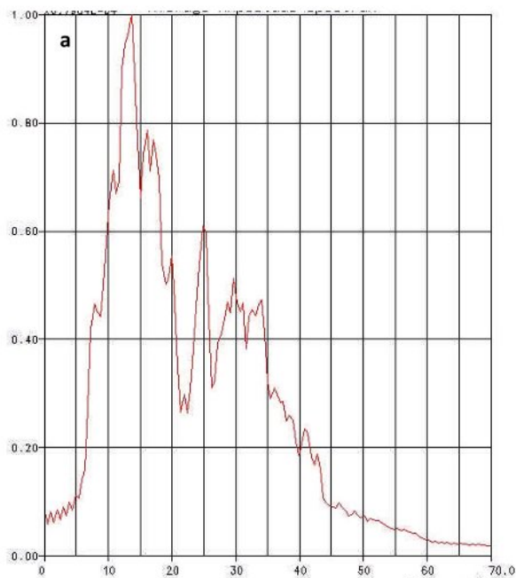
▲ Рис. 5. Сопоставление спектров отражённых волн, зарегистрированных с использованием группы 2-х вибраторов на базе 10 м и 3-х вибраторов на базе 20 м (ПР1, ПВ1051, \Delta F=6-60 Гц, T=24 с, \text{пнак}=6 , начальный скос 200 мс., конечный скос 500 мс., окно анализа 1,5-2,5 с, вне конуса доминирующих поверхностных помех); а – два вибратора на базе 10 м; б – три вибратора на базе 20 м
