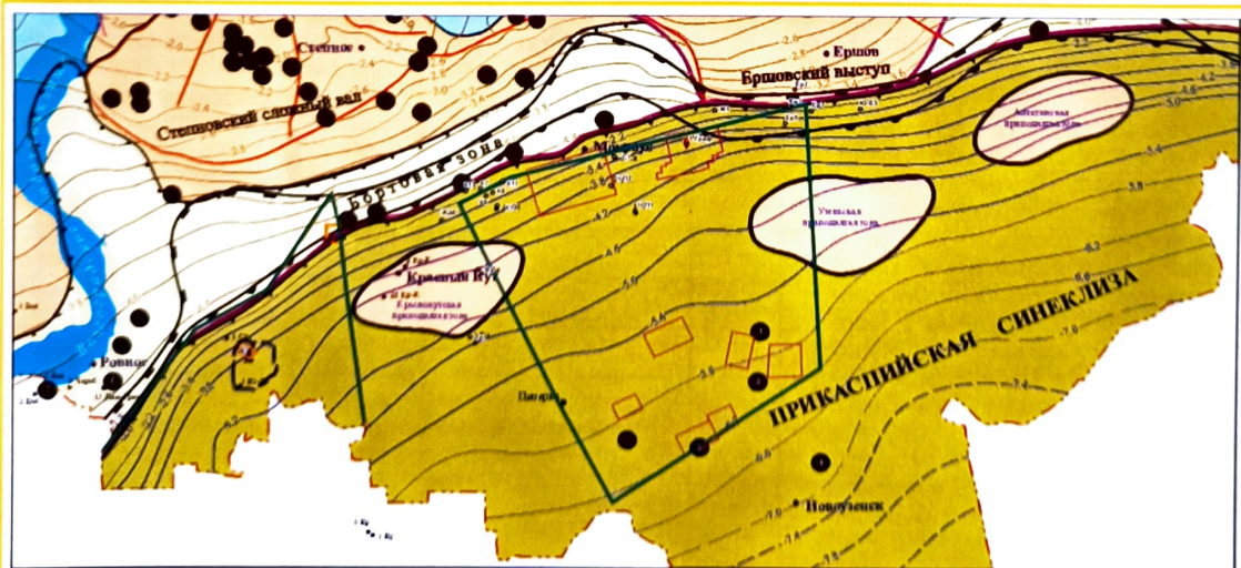
1 - контур Прикаспийского лицензионного участка, 2 - контур сейсмических работ МОГТ-3Д, 3 - контур центральной части среднефранской карбонатной базиса, 4 - контур среднефранской рифогенной постройки, 5 - границы структур I порядка, 6 - границы структур II порядка, 7 - седиментационные уступы (а - московско-артицкий, б - верхнеивановско-нижнебашкирский, в - фаменско-нижнеуральский, г - средне-верхне-франский), 8 - месторождения УВ (1 - Таловское, 2 - Старинское, 3 - Куриловское, 4 - Спортивное, 5 - Узеньское, 6 - Лиманно-Грачевское, 7 - Белокаменное), 9 - изогипсы по подошве кузнецких отложений, в км, 10 - изогипсы по подошве саргавских отложений, в км, 11 - скважины
